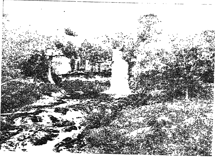
(अ) थॉर्नटन फोर्स, इंग्लैटन, यौर्कशायर—कोयला युग की चूने की चट्टानों के सिचीलीनिया भाग के स्तर के झरन ।
